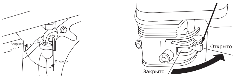
Рис. 14. Топливный кран
